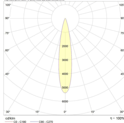
*Albi 7W/13W/18W 15°
