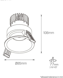
Albi Maxi Adjustable 7W
