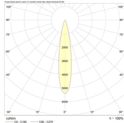
*Albi 7W/13W/18W 15°
