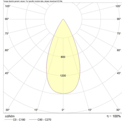
*Bron 7W/13W/18W 50°
