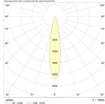
*Bron 7W/13W/18W 15°
